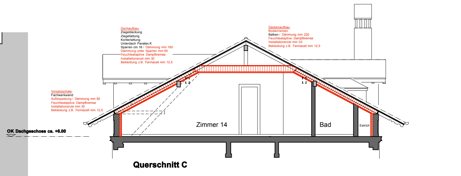
Schnitt C
