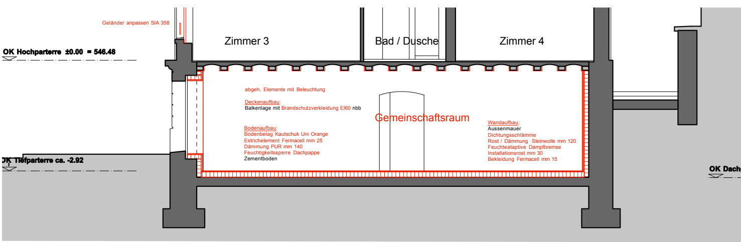
Schnitt D
